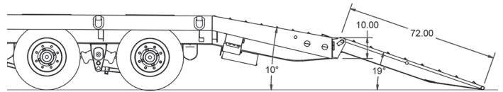
5' Beavertail w / 6' Air Ramp
